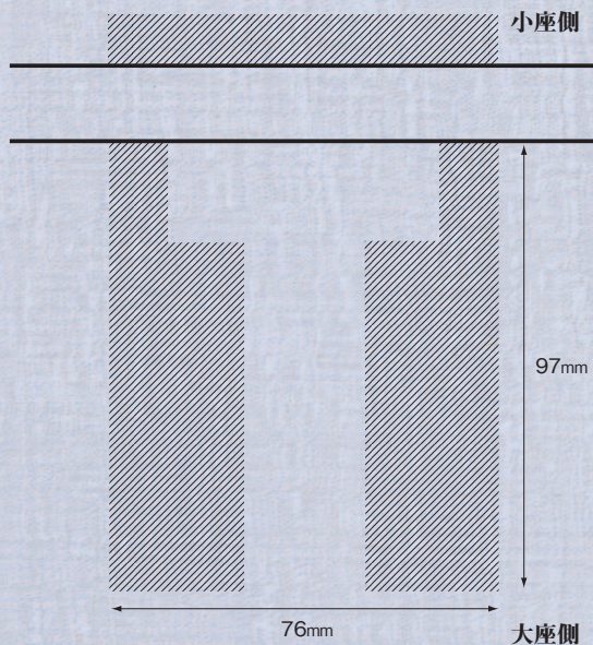
大座・小座
