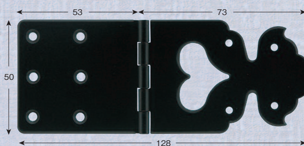
古代透民芸平丁双
